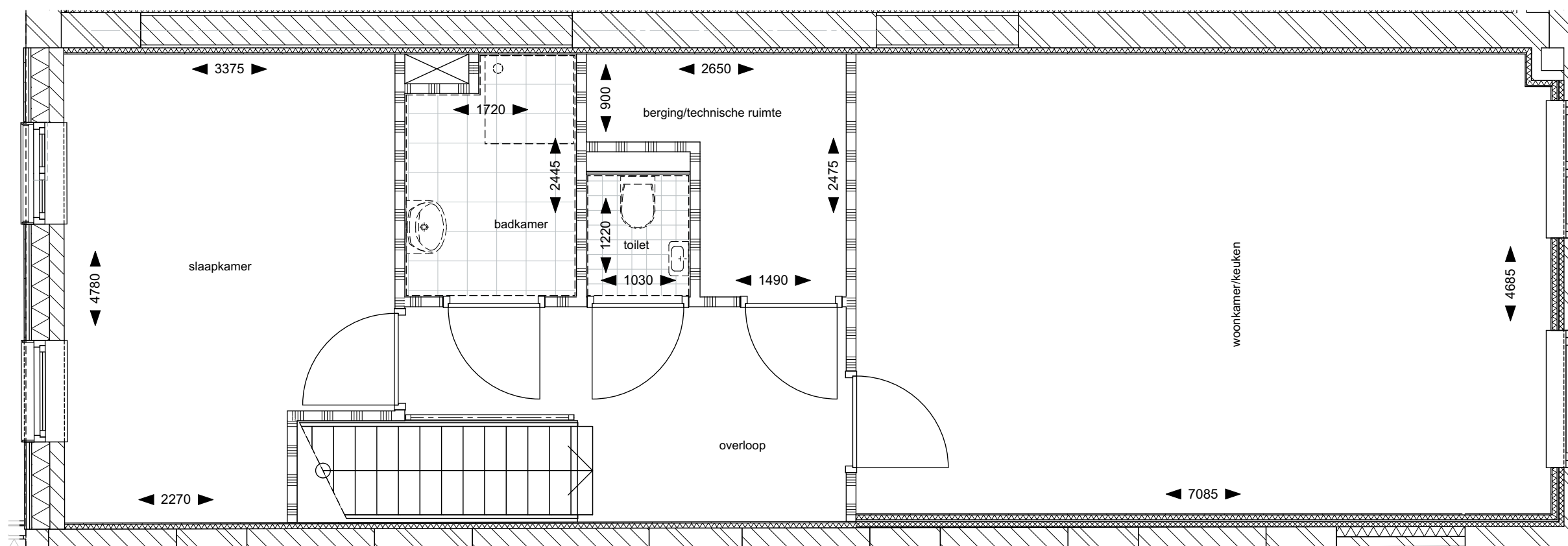
1e verdieping 3750+
