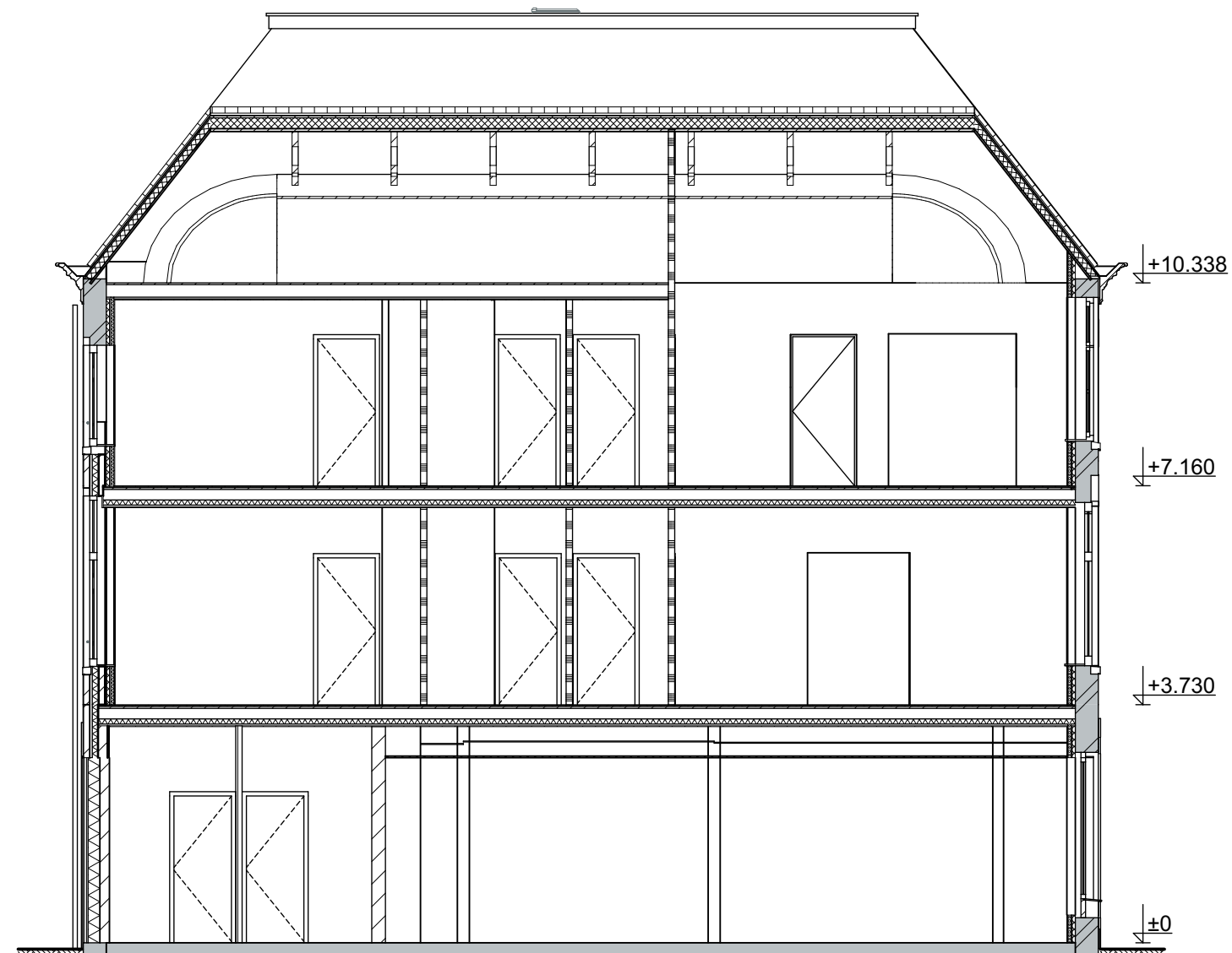
doorsnede bnr 35 en 37
