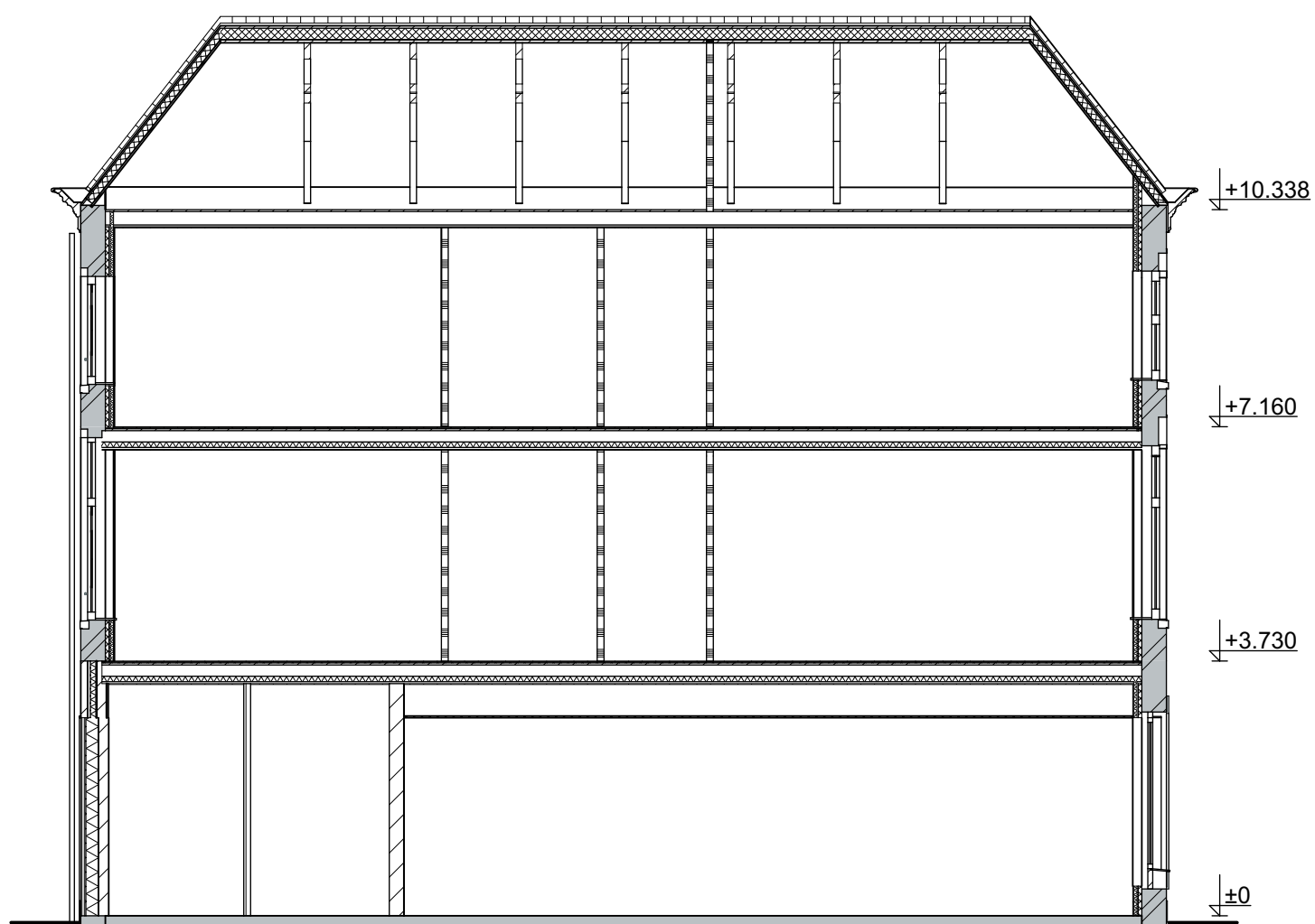
doorsnede bnr 36 en 38
