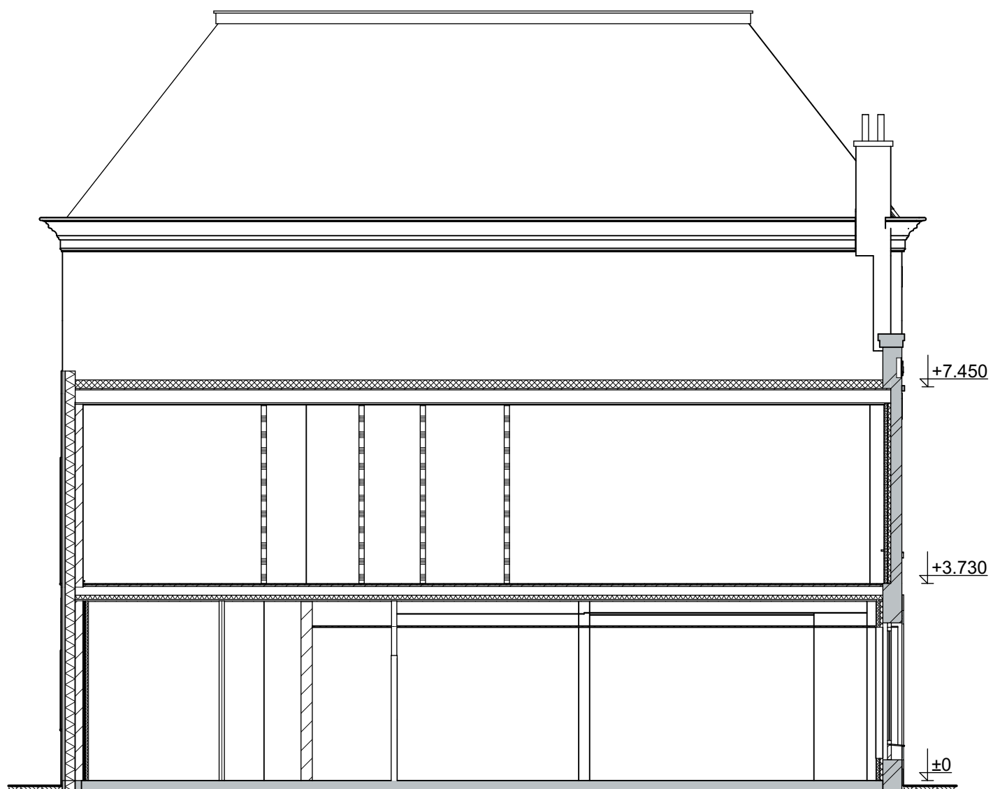
doorsnede bnr 34
