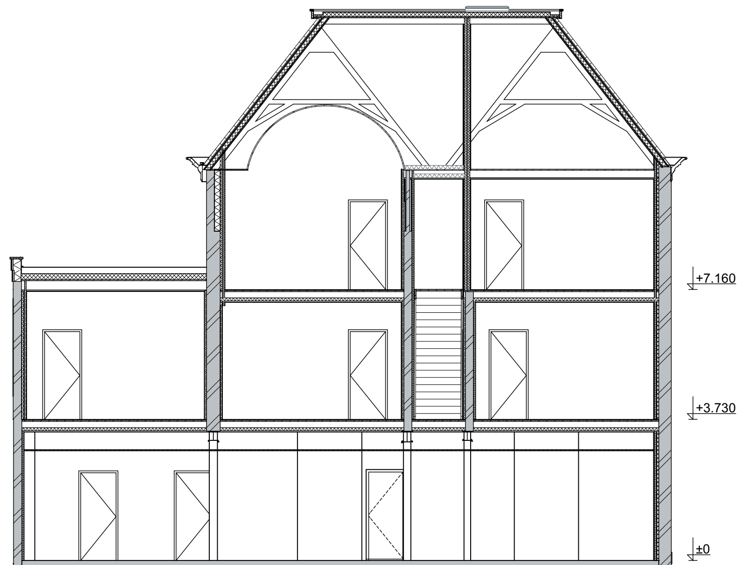
doorsnede bnr 34, 35, 36, 37 en 38
